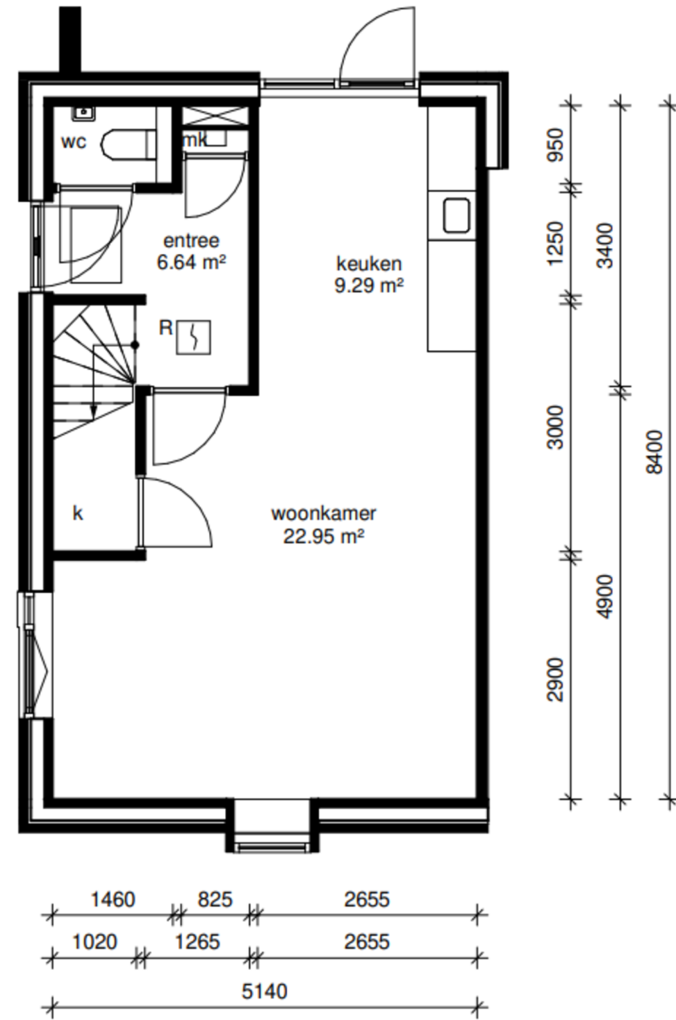
begane grond
